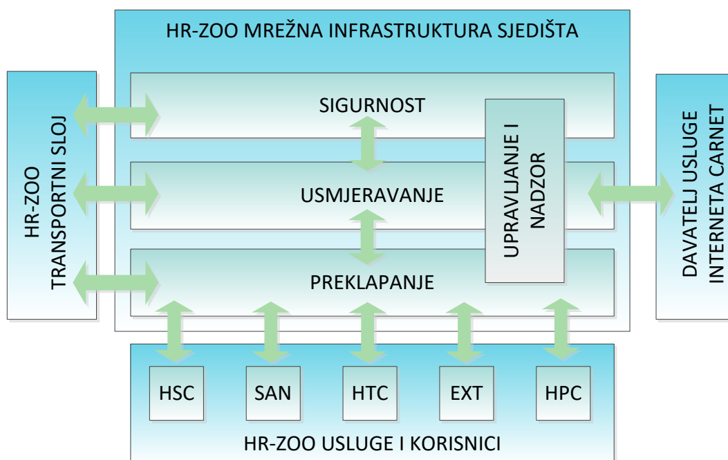
Slika 2: Pregled DC LAN-a
