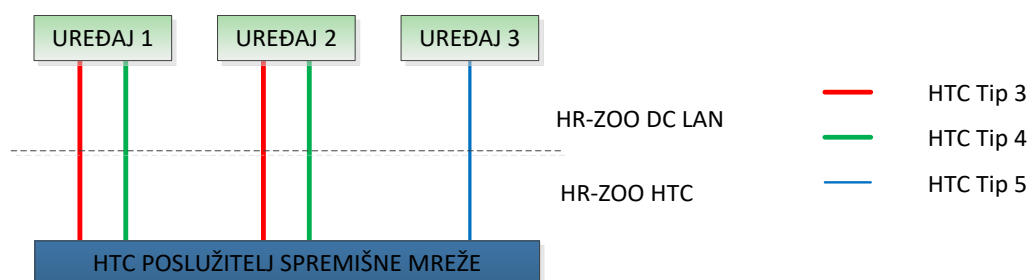
Slika 8: Povezivanje HTC fizičkog poslužitelja za brzo spremište
