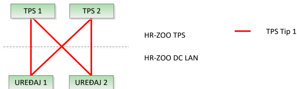
Slika 13: Povezivanje na HR-ZOO transportni sloj
