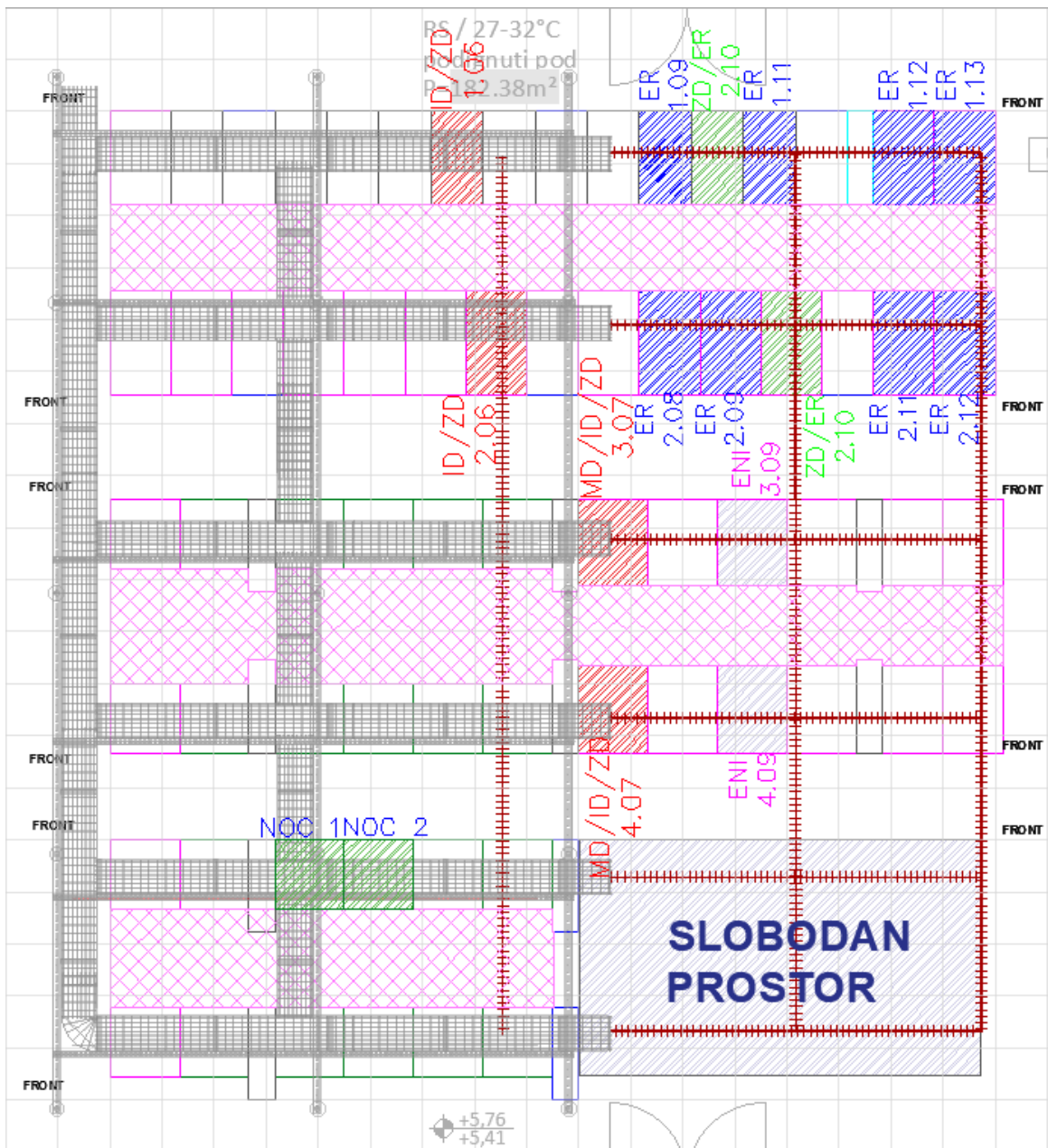
Slika 16: HR-ZOO ZG1 prostorni nacrt kabljskih trasa 2.kat - situacija
