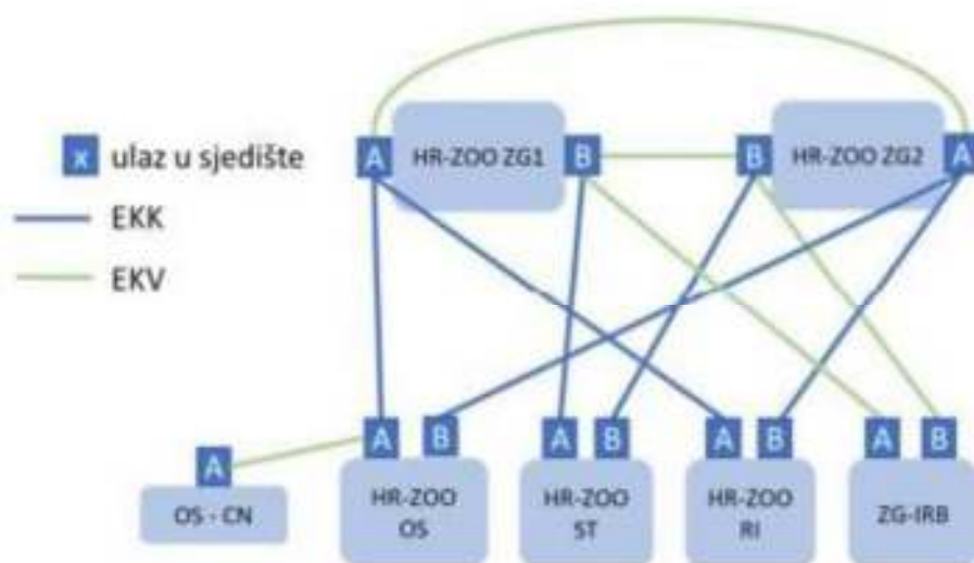
Slika 1. Fizička topologija
